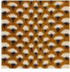
L3914_LES_EC AILLES_C516_C 531_FE
